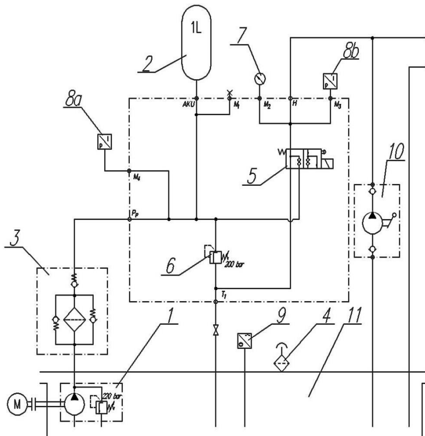
Rys. 6. Schemat ideowy agregatu hamulcowego HAH 1 [1]
